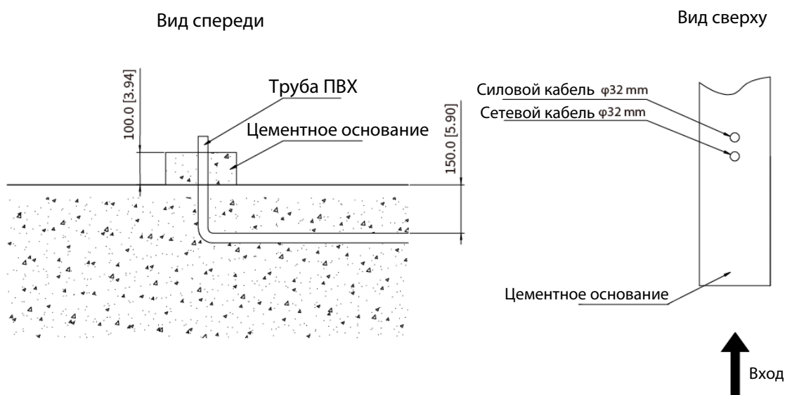
Рисунок 2-2. Схема подключения
