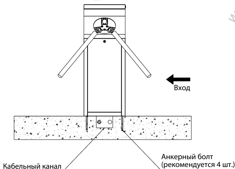
Рисунок 2-6. Кабельный канал
