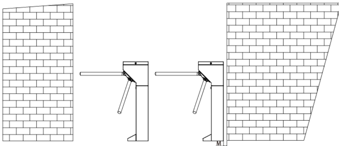
Рисунок 2-3. Требования к расстоянию
