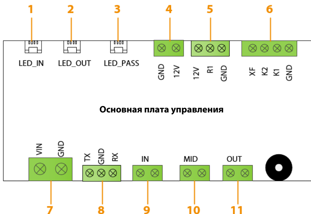
Рисунок 2-8. Основная плата управления
