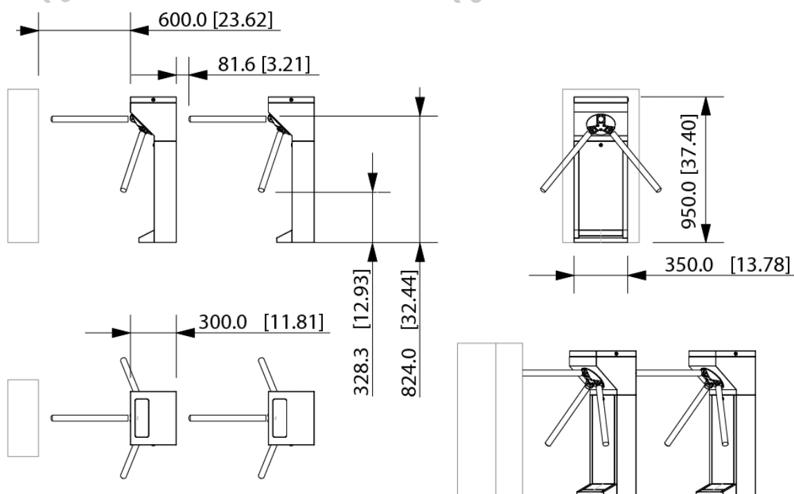
Рисунок 1-1 Габаритные размеры (единица измерения: мм [дюйм])
