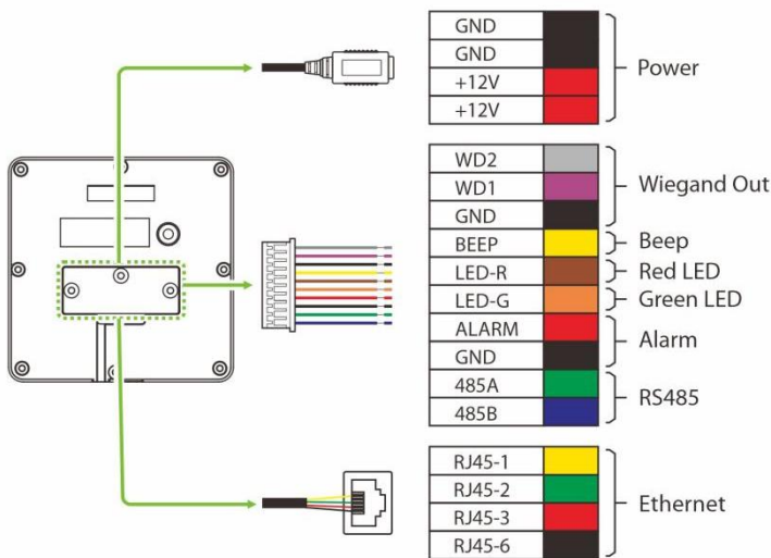
Рисунок 1-2: Описание клемм
